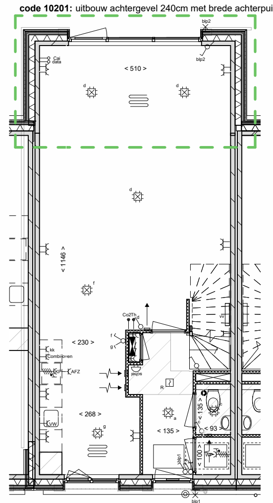
begane grond
