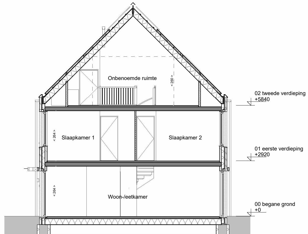
doorsnede
