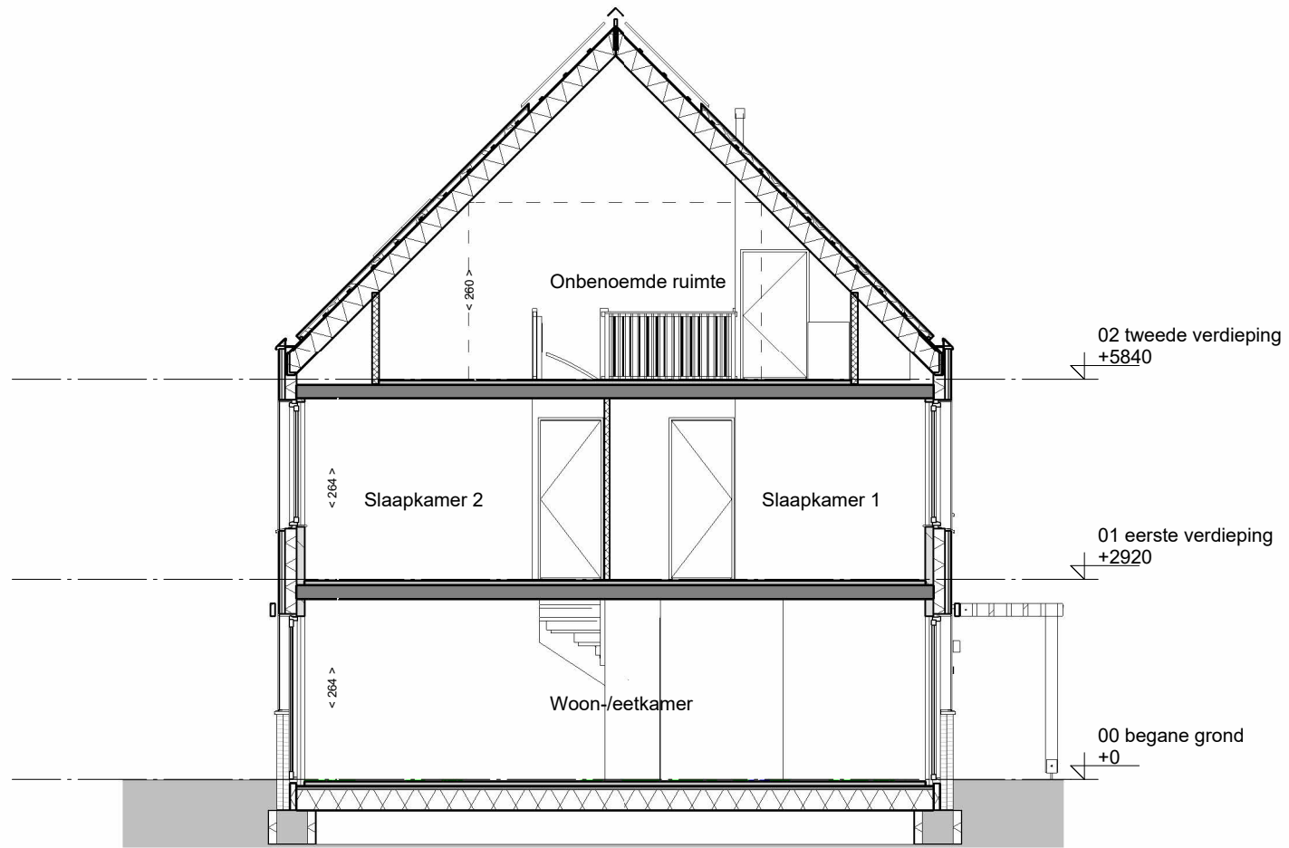
doorsnede
