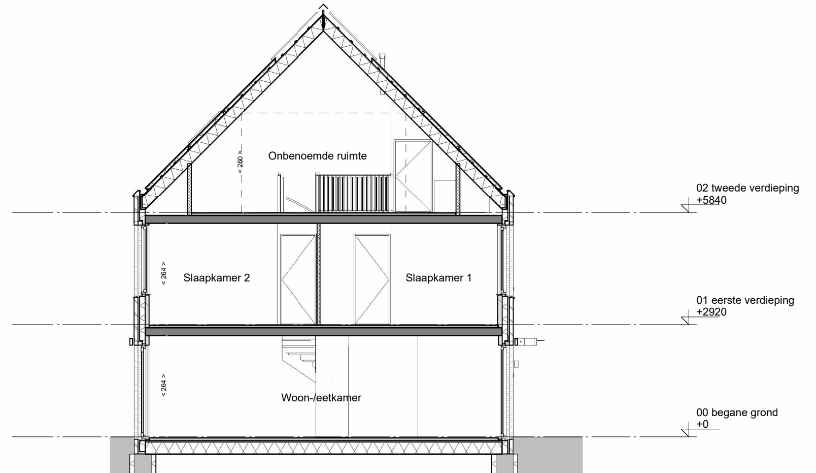
doorsnede
