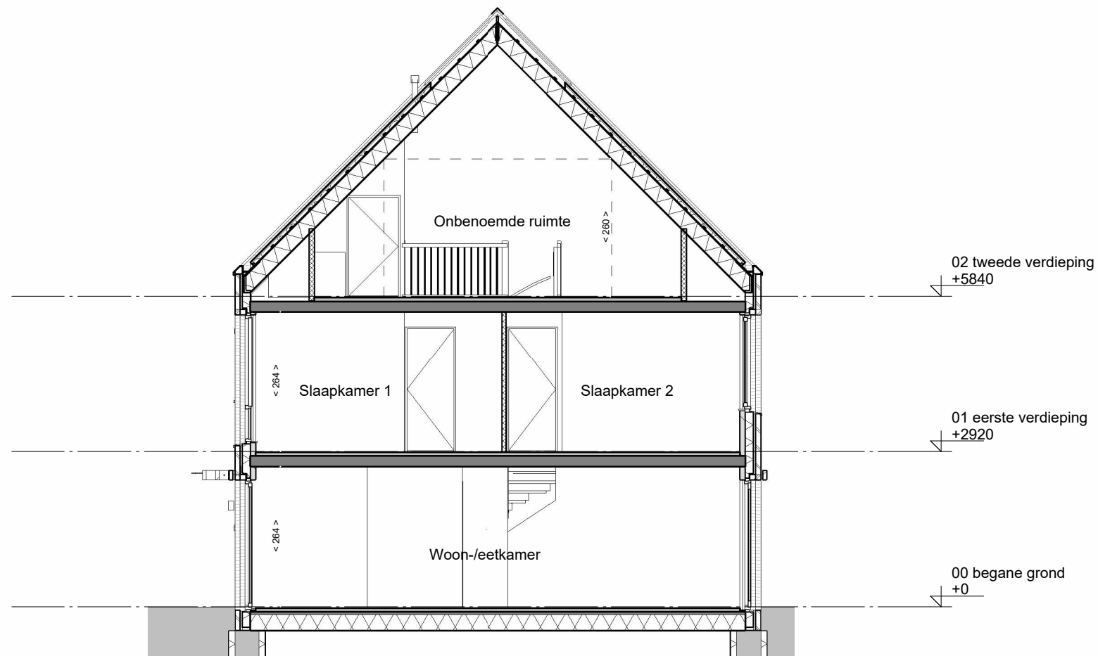
doorsnede
