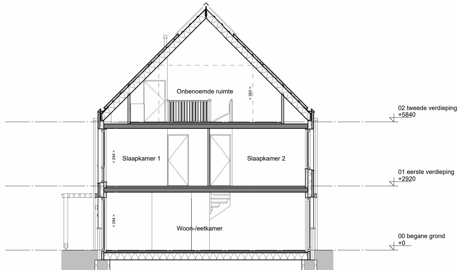
doorsnede
