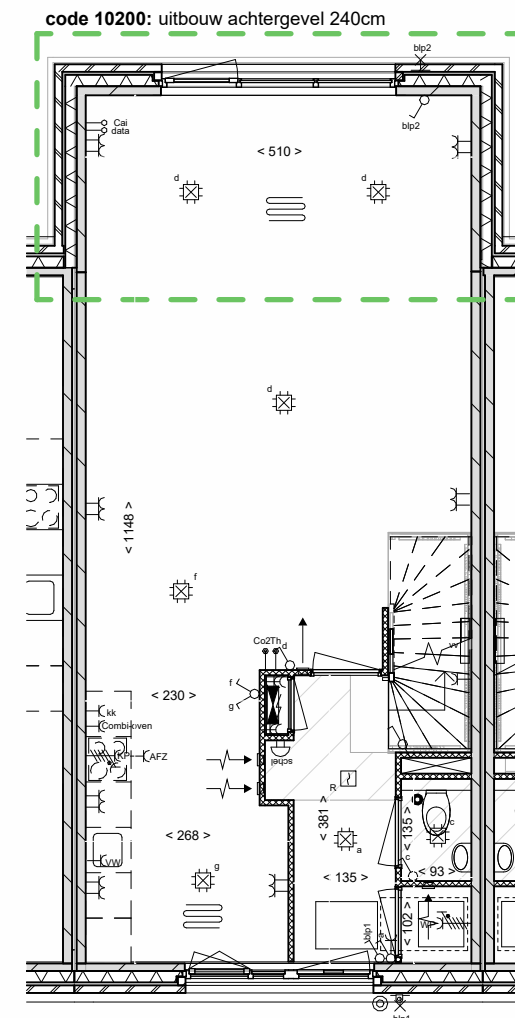
begane grond
