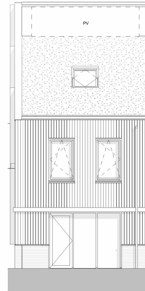
achtergevel
