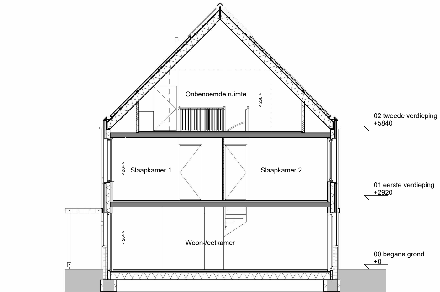
doorsnede
