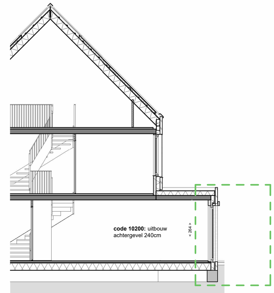
doorsnede
