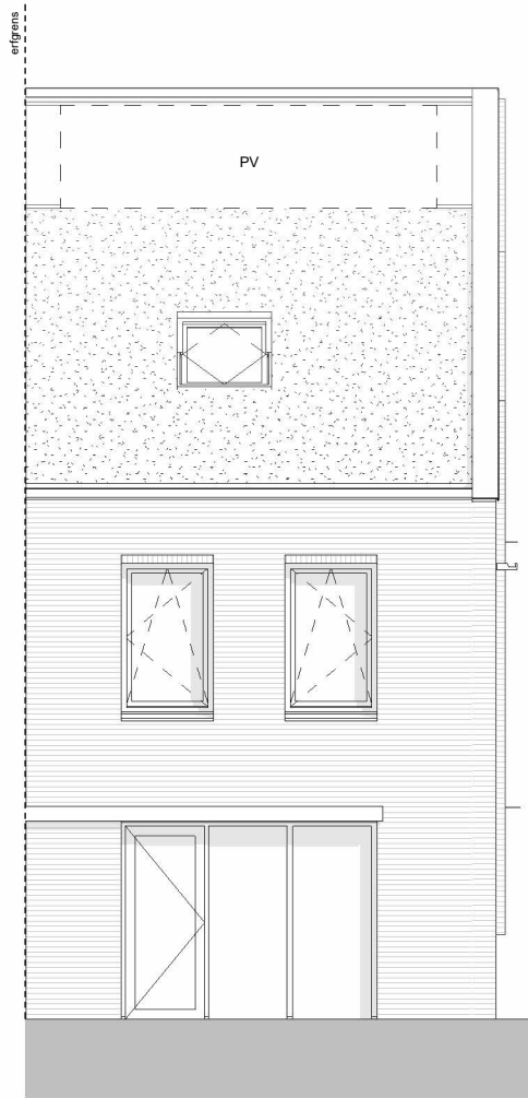
achtergevel
