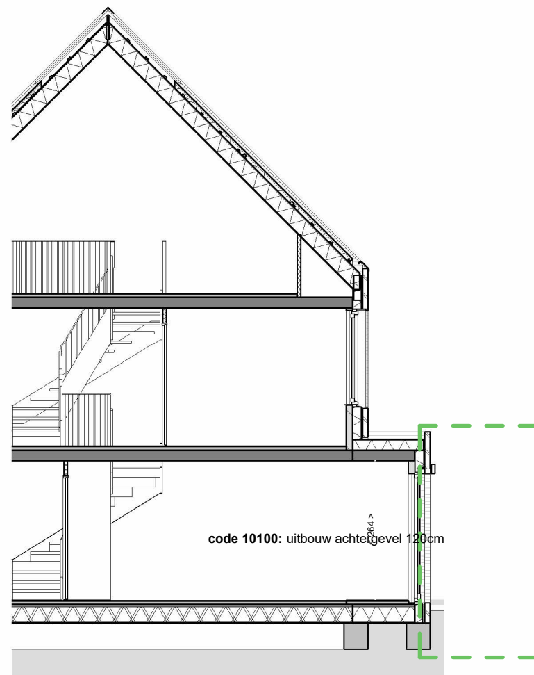
doorsnede
