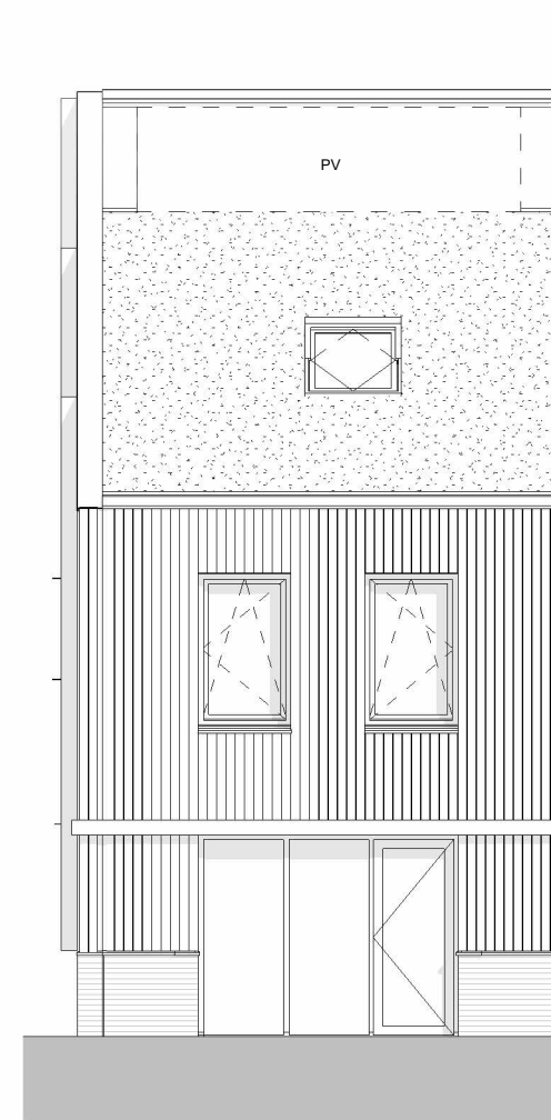
achtergevel
