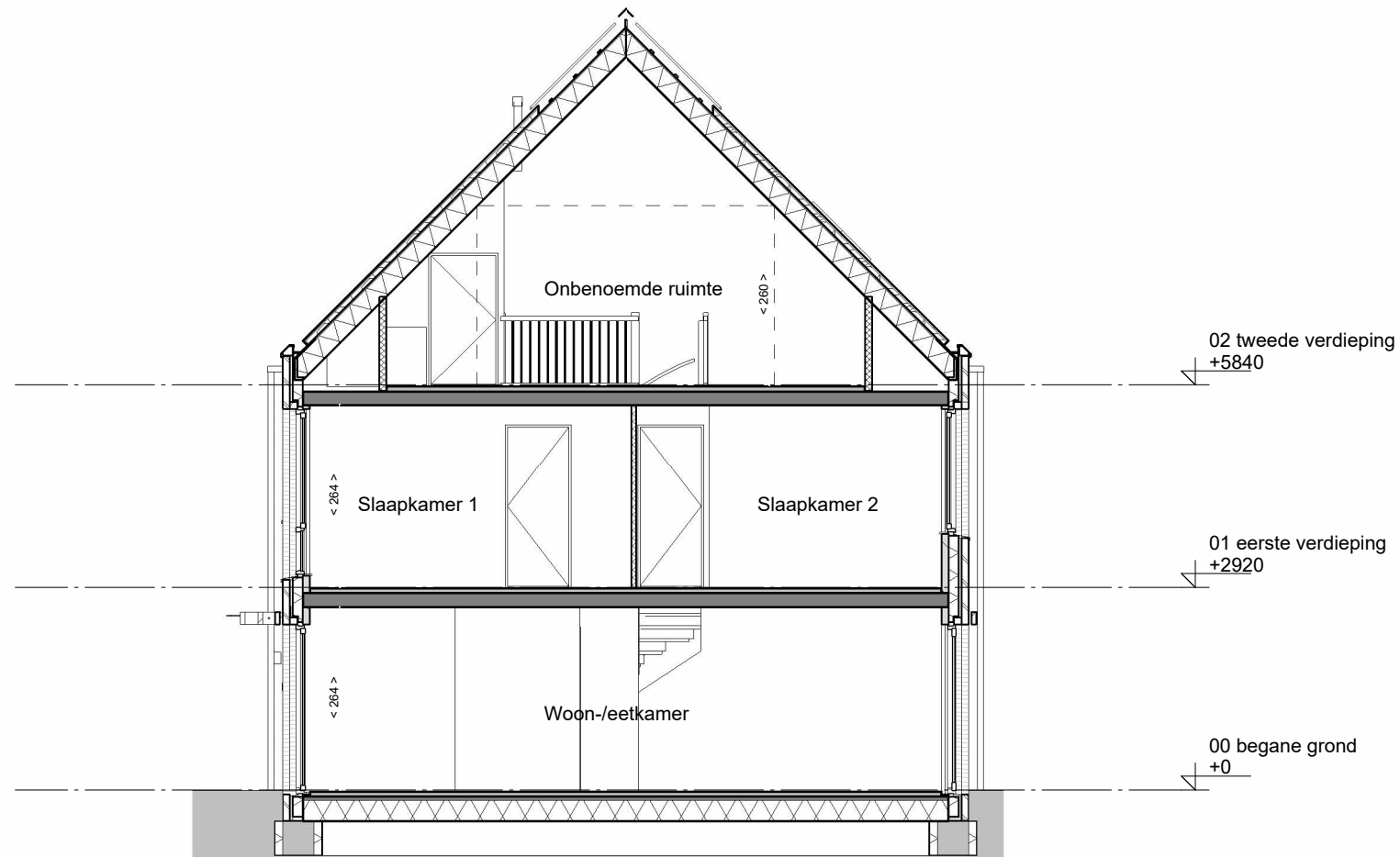
doorsnede
