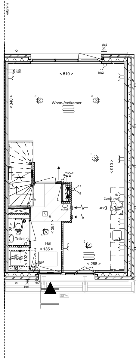
begane grond
