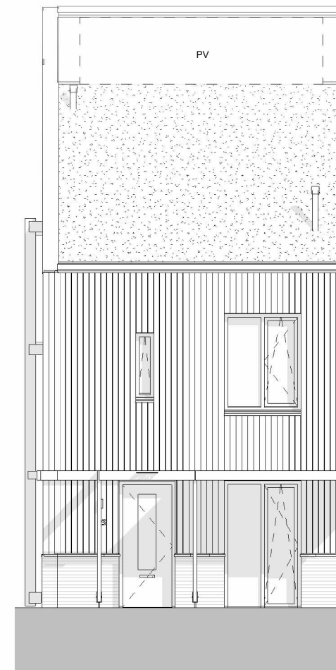
voorgevel
