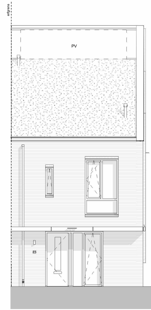
voorgevel
