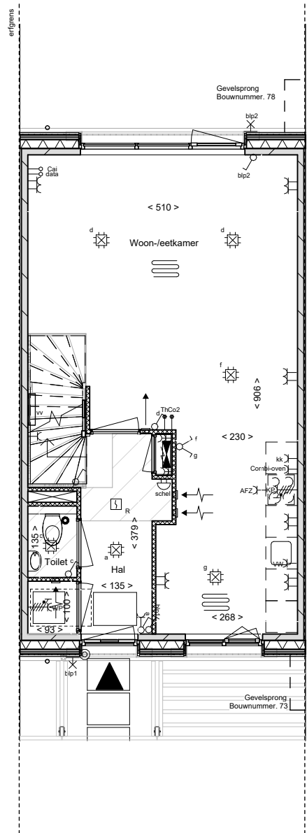
begane grond
