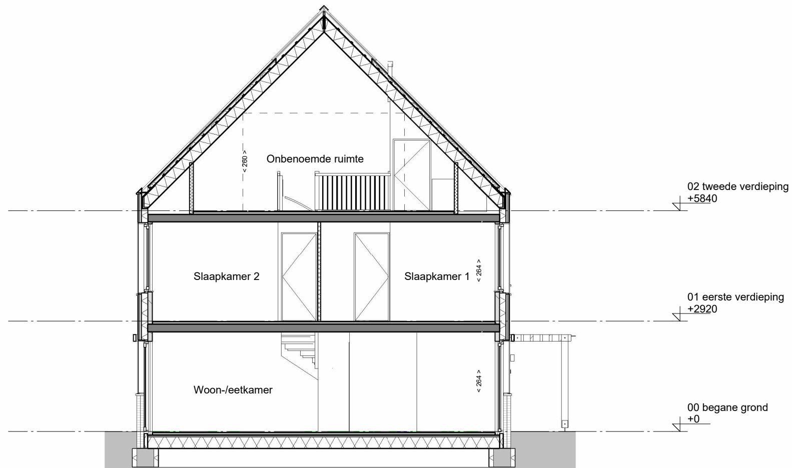
doorsnede
