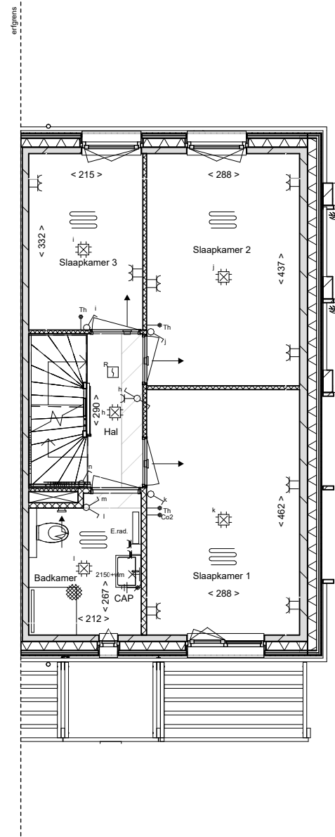
eerste verdieping
