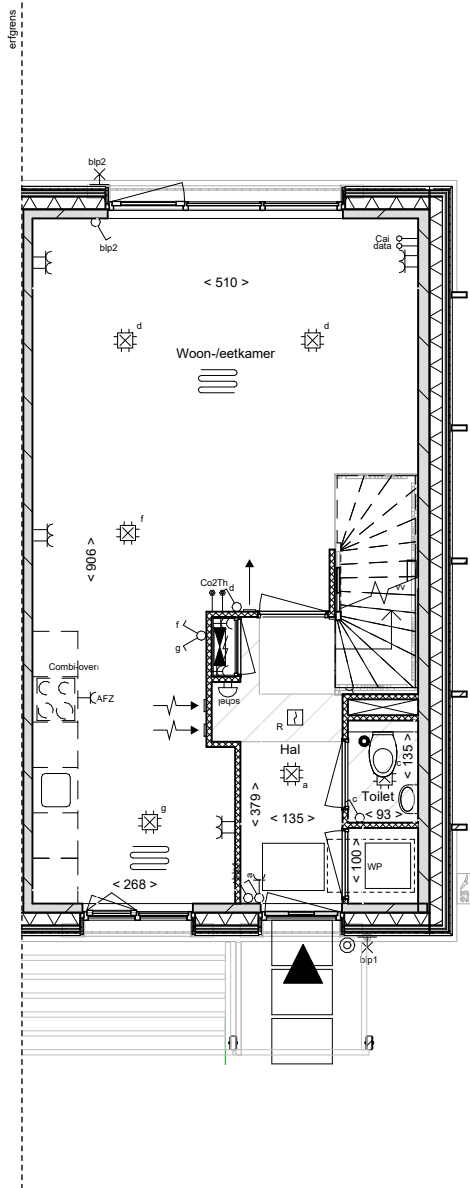
begane grond
