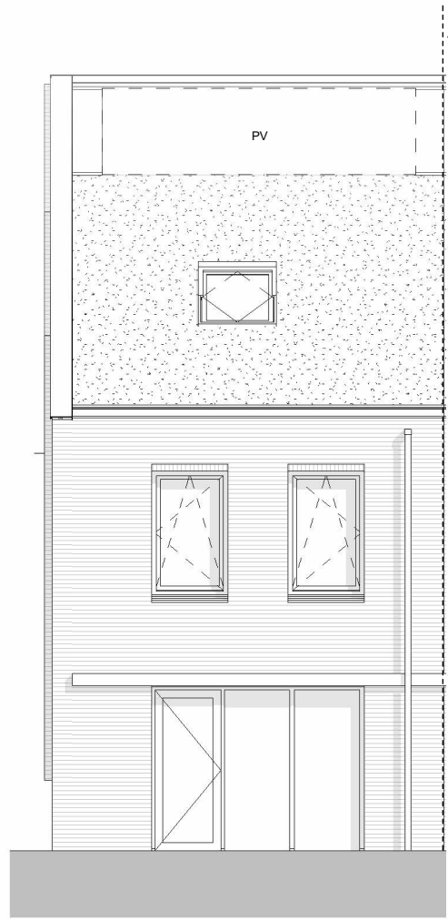
achtergevel
