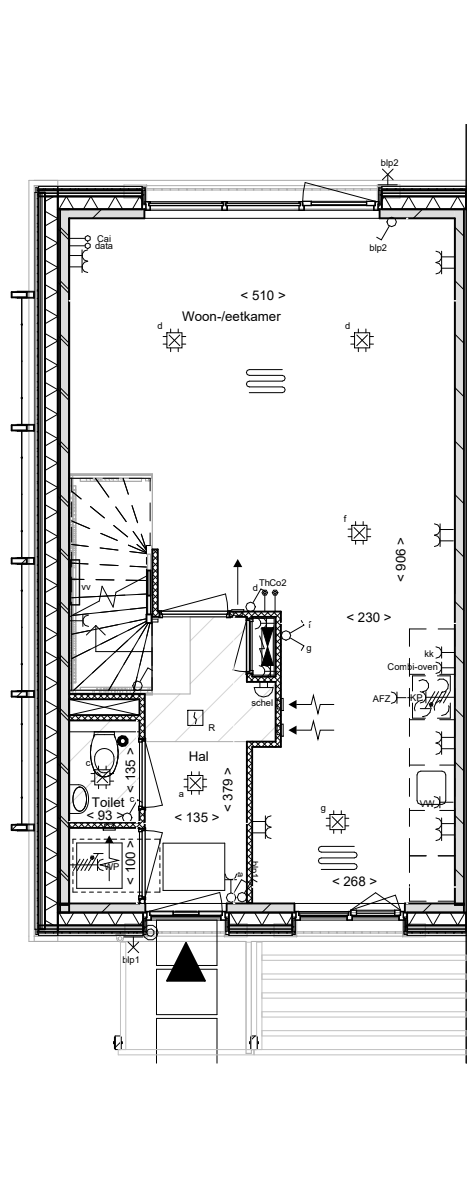
begane grond
