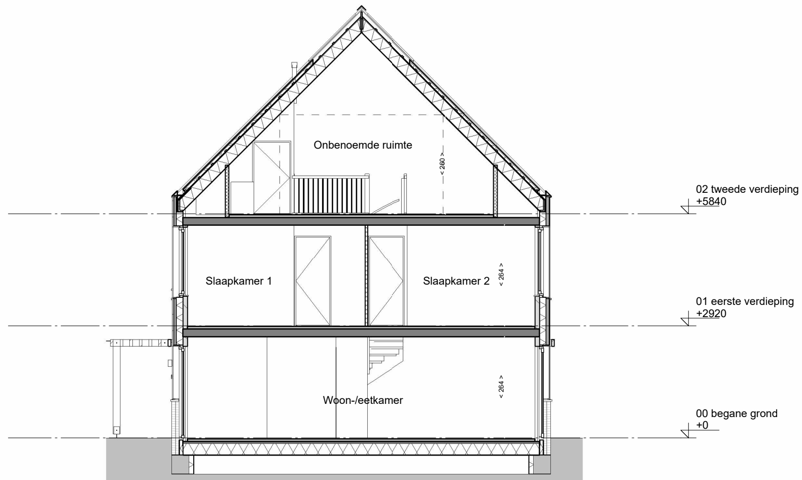
doorsnede
