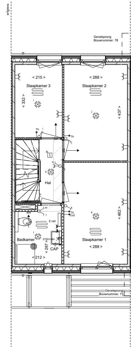
eerste verdieping
