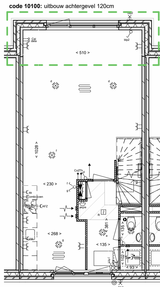
begane grond
