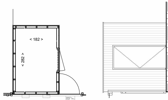
Begane grond
